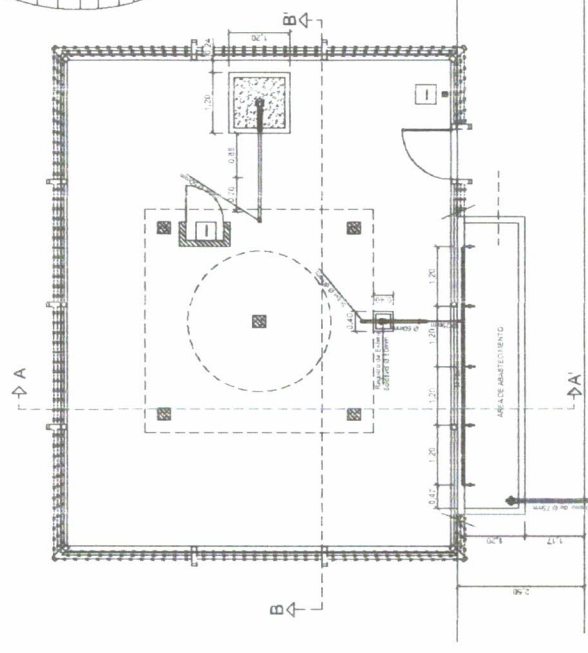
PLANTA BAIXA - INSTALAÇÕES ÁGUA FRIA ES: 108
